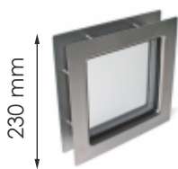
Okno nr: 2435R1
